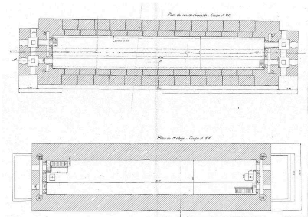
Plan d'une poudrière de la vallée de Kerhuon, signé de l'ingénieur en chef Fille, commandant de la Pyrotechnie, 5 décembre 1940 : rez-de-chaussée et étage
