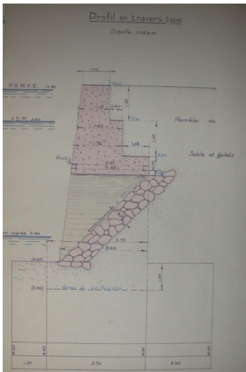
Plan du nouveau quai : profil en travers type, 1931 (AD 22)
