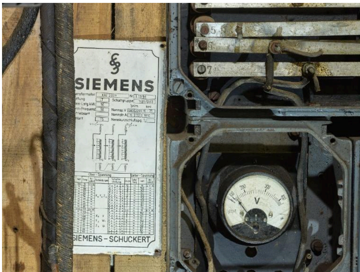
Vue intérieure : salle des machines pour deux groupes électrogènes, détail du tableau électrique de la batterie antiaérienne Rossitten. A gauche, plaque constructeur Siemens-Schuckert
