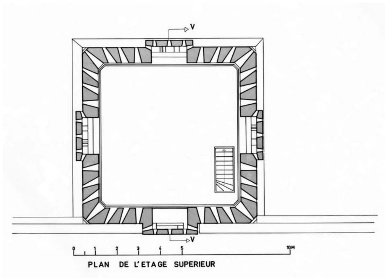
Plan de la terrasse de la tour-modèle n° 3 du Toulinguet, Camaret-sur-Mer
