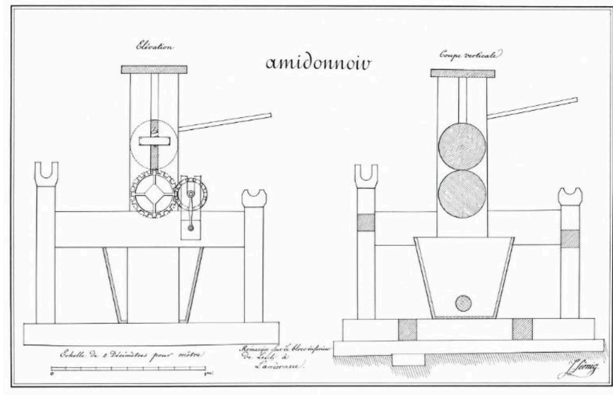
Amidonnoir. Elévation et coupe verticale. Dessin généré par l'IA, d'après un dessin original de Joseph-Guillaume Sénez (Lin et chanvre en Bretagne)
