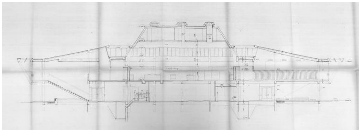
Réfectoire - cuisine, coupe transversale (de la partie centrale, selon un axe ouest-est), Louis Arretche, architecte, 1961.
