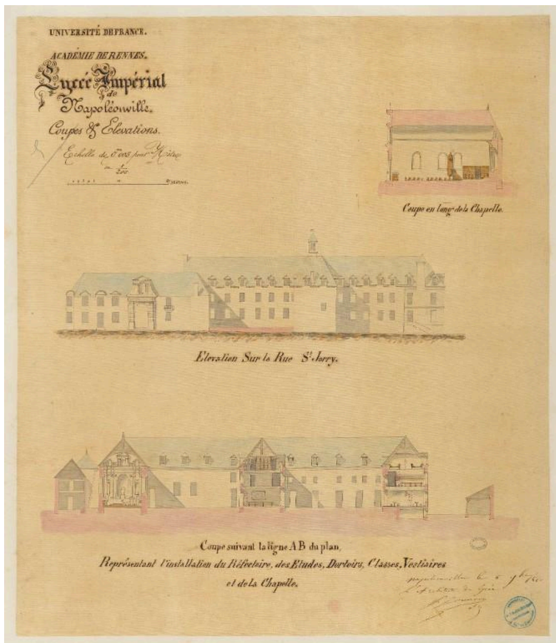
Lycée impérial de Napoléonville. Coupes et élévations. 1842.
