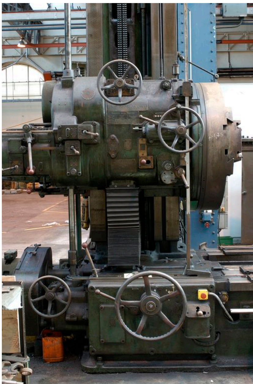
Vue de la halle d'usinage : aléseuse Malf Richard (1948), détail des volants
