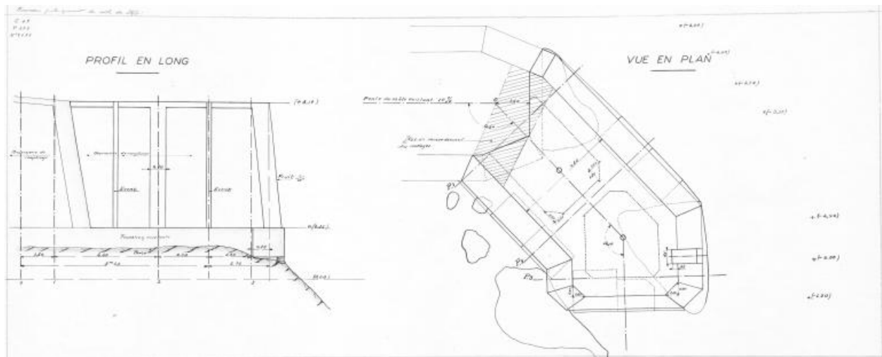
Plan et profil du second prolongement du môle (non daté)
