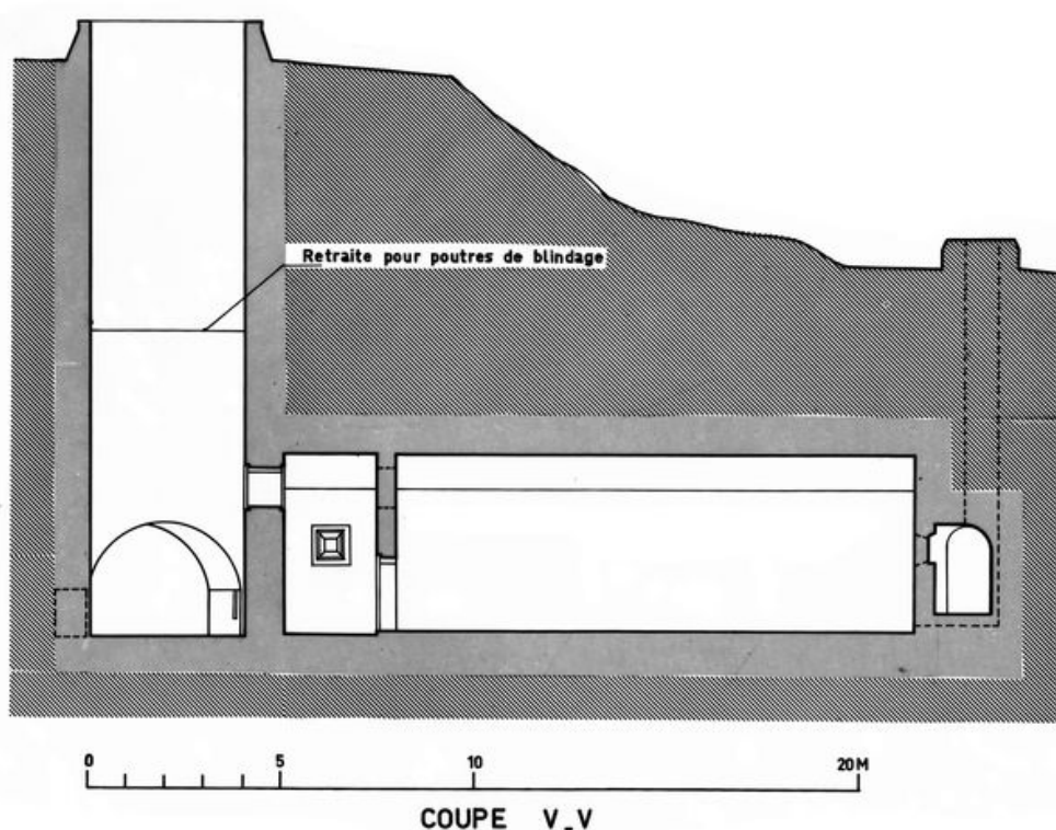
Coupe du magasin à poudre sud (Lecoq)
