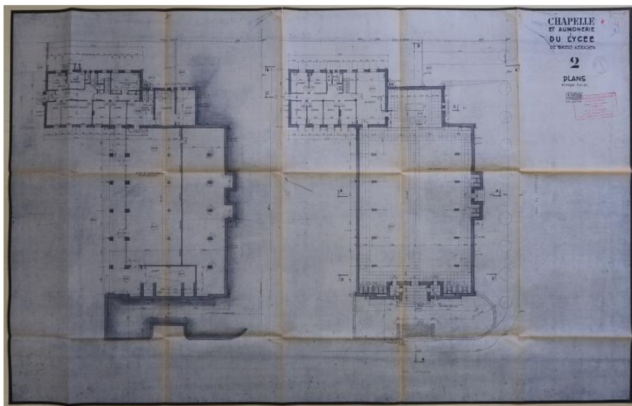
Chapelle et aumônerie du lycée. Plans. Jean-Baptiste Mathon, architecte, 28.5.58.
