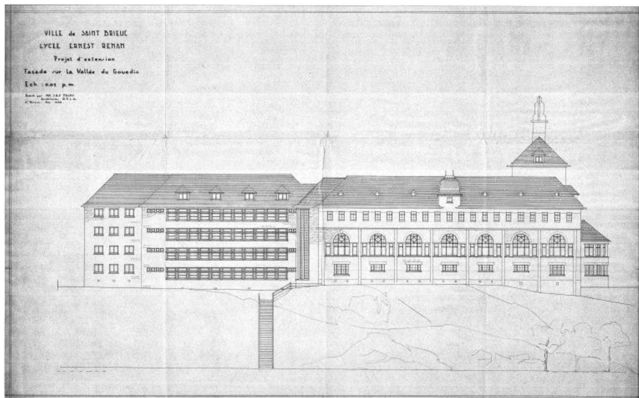
Façade sur la vallée du Gouédic, mai 1959. Jean et Yann Fauny, architectes.
