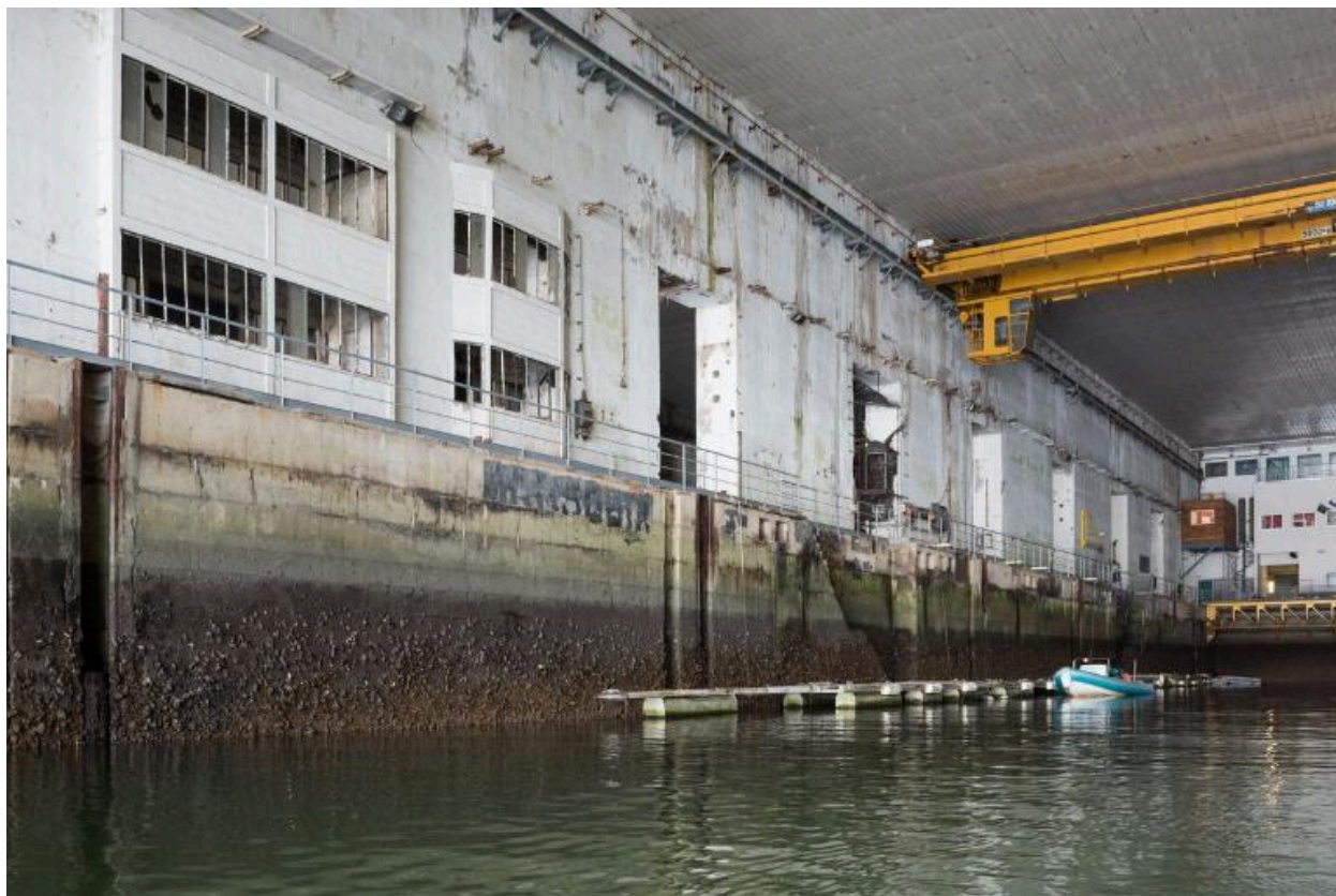
Vue de l'alvéole D en eau : quai n° 20 et salles des pompes aménagées dans l'épaisseur du mur de refend entre les alvéoles C et D
