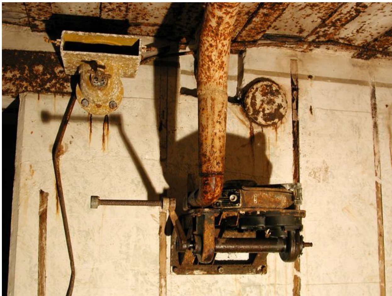
Vue du ventilateur (modèle HES de 2,4 m3 pouvant fonctionner avec deux manivelles)
