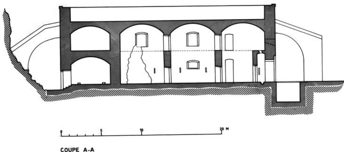
Coupe A-A de la caserne défensive
