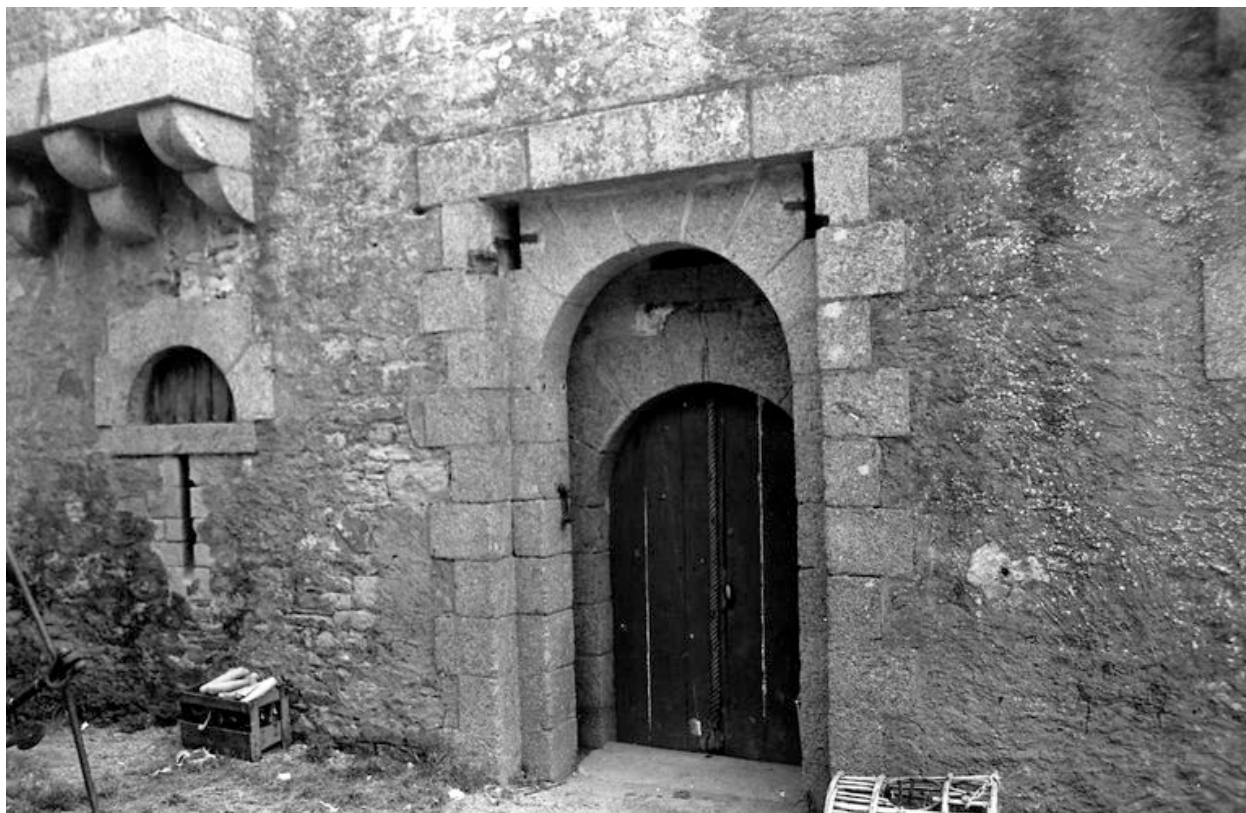
Vue du corps de garde crénelé n° 3 du bourg de Roscanvel en 1969 : porte d'entrée. A noter : la feuillure d'encastrement du pont-levis et le passage des chaînes de manoeuvre
