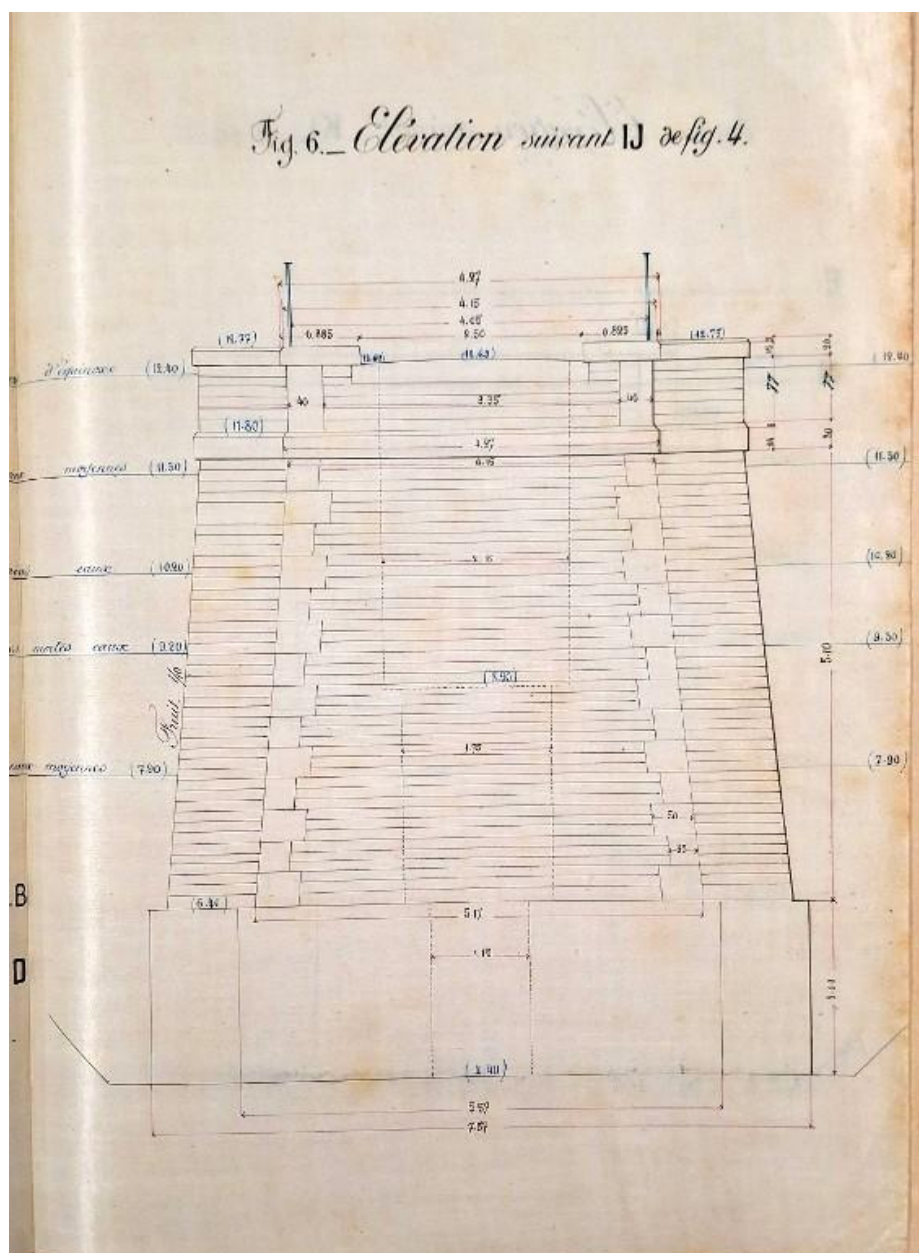
Dessin de la culée rive droite (9 octobre 1891)
