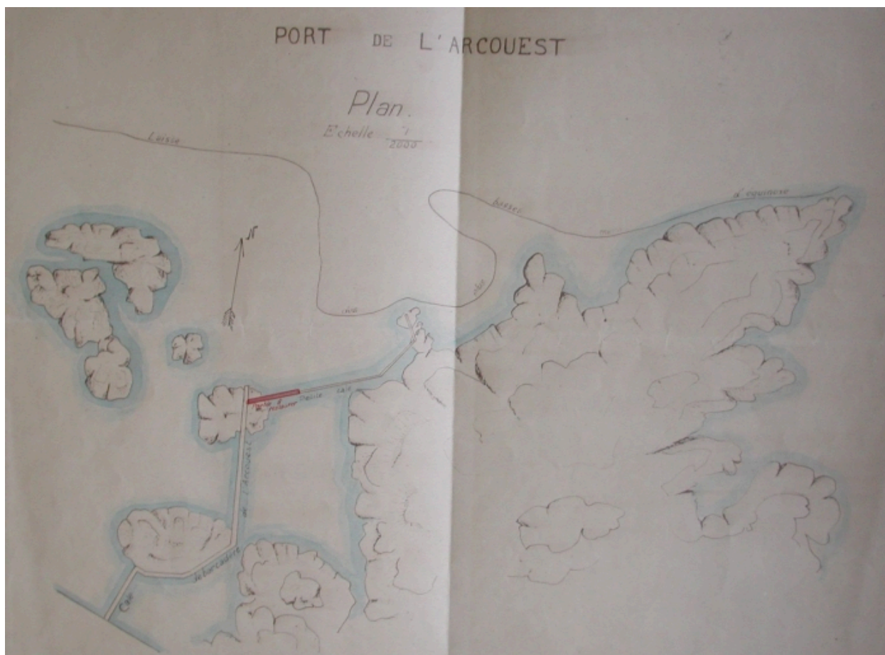
Plan général des cales de l'Arcouët, projet de restauration de la petite cale, 1923 (AD 22)
