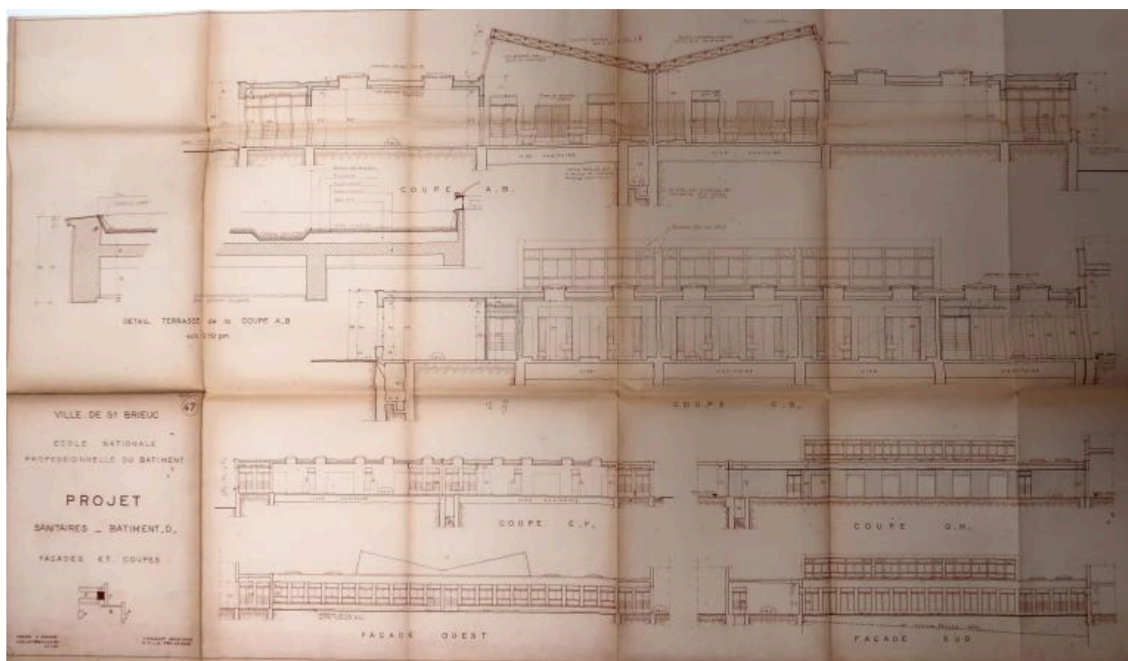
Sanitaires - Bâtiment D. Façades et coupes. Yves Moignet, architecte, 1960.
