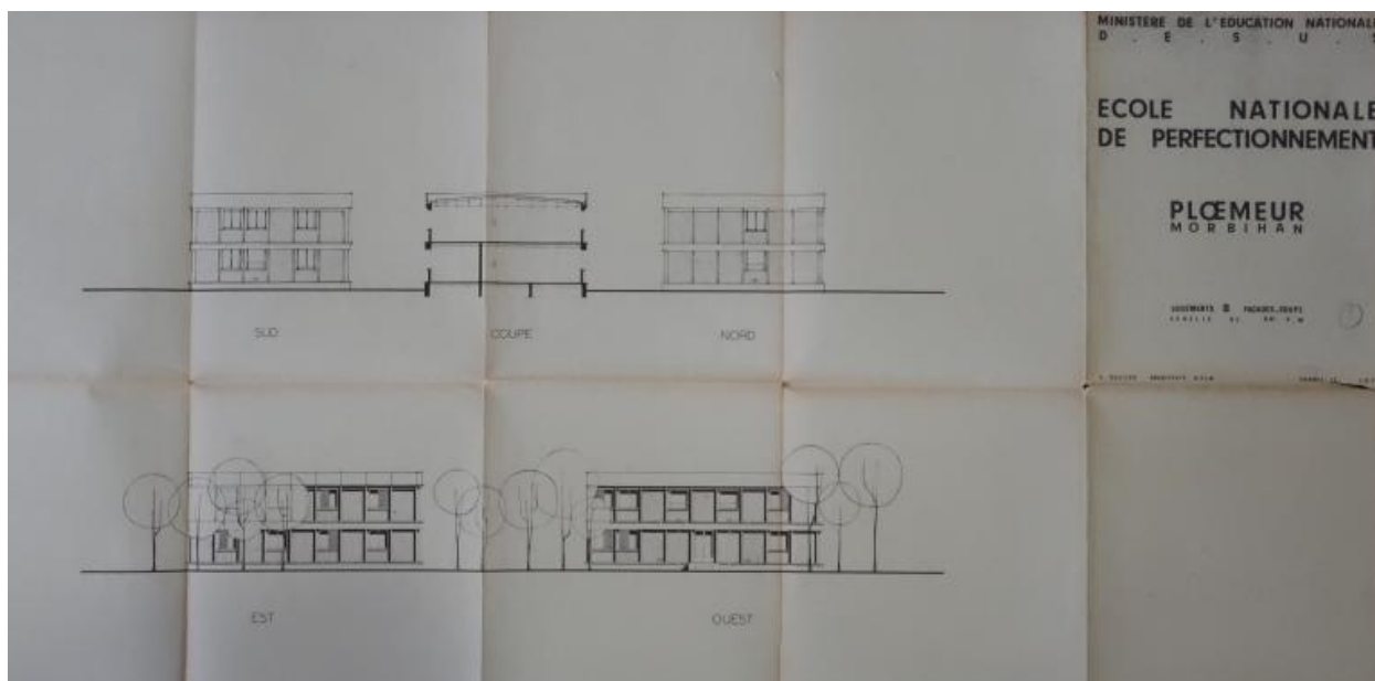
Logements B, façades - coupe. Yves Guillou, architecte, 1967.
