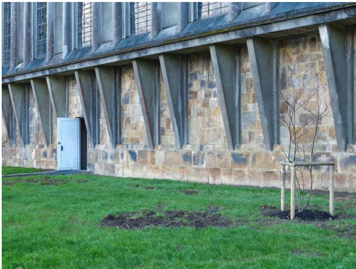
Eglise Saint-Louis, parement en pierre de Logonna, structure béton, mur ouest
