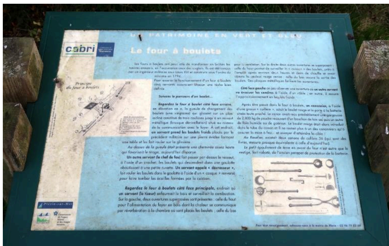
Principe de fonctionnement du four à boulets (signalétique en place réalisée d'après les travaux de Guy de Sallier Dupin)
