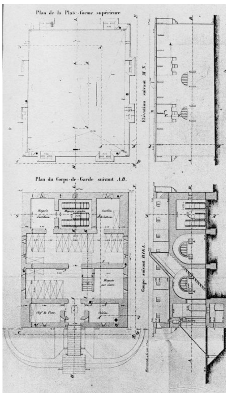
Plans, coupes, et élévations des réduits de batteries : corps de garde crénelé n° 3 pour 20 hommes servant de réduit à une batterie de 4 pièces, 1846, détail
