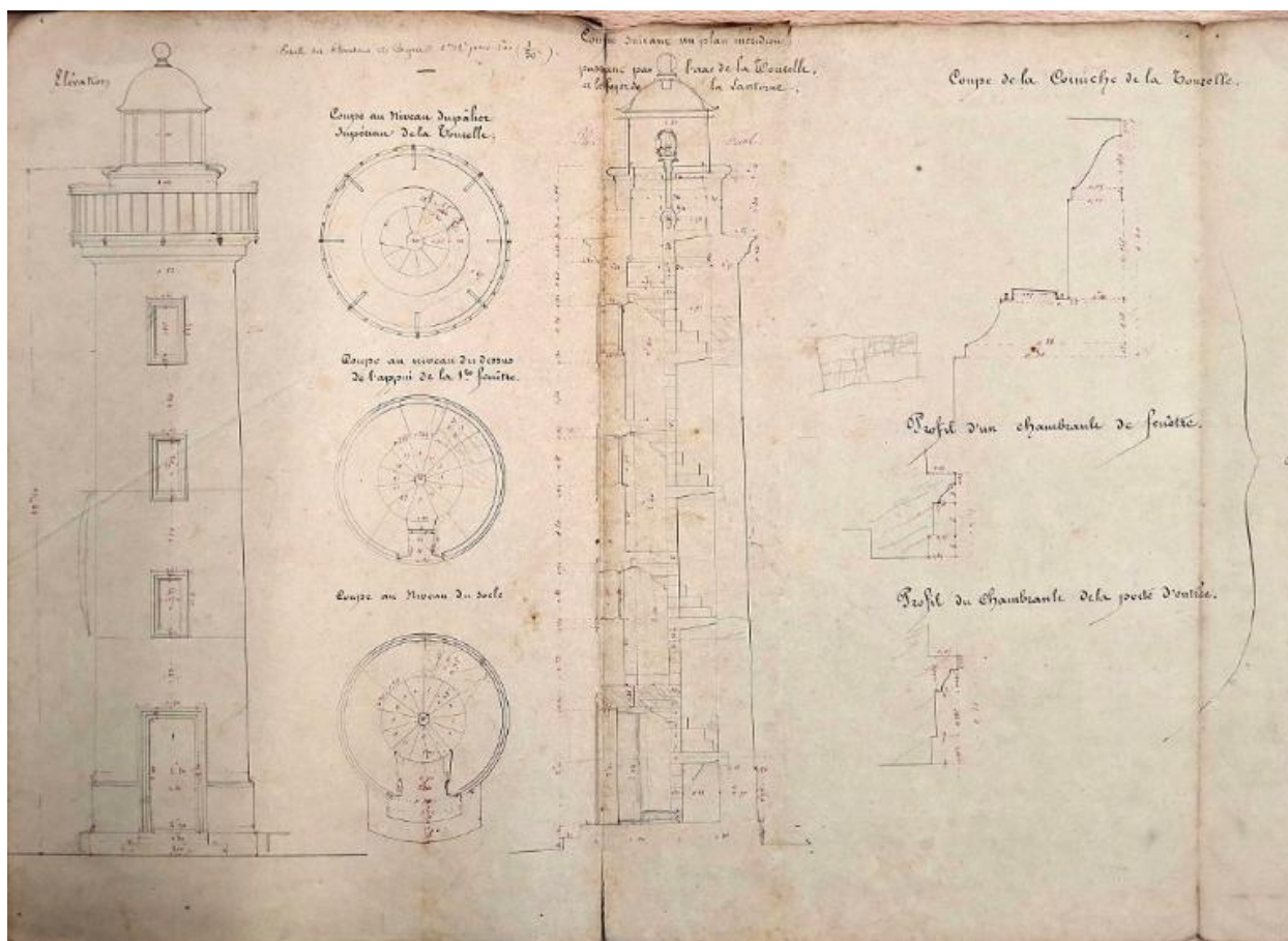
Elévation, coupe et profil du phare de la pointe de l'Aigle (29 novembre 1851)
