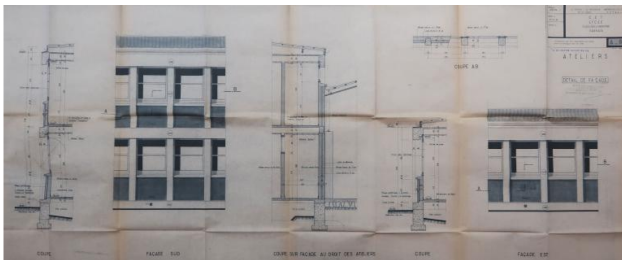
Ateliers, détail de façade. Hervé Péron et Alexandre Weisbein, architectes, 1964.
