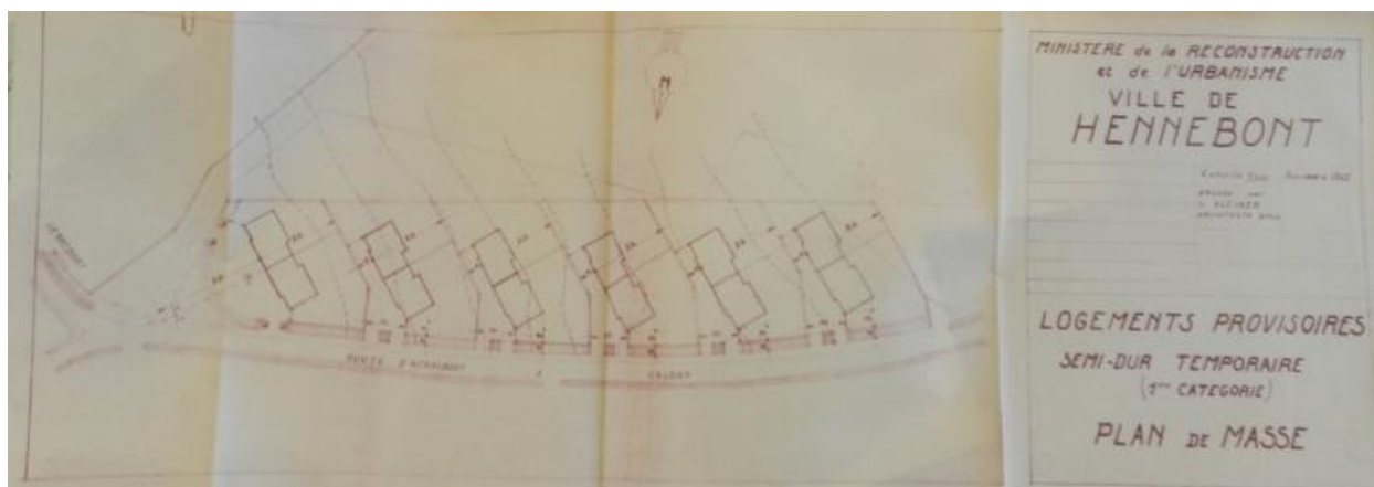
Plan de masse des logements provisoires semi-dur temporaire
