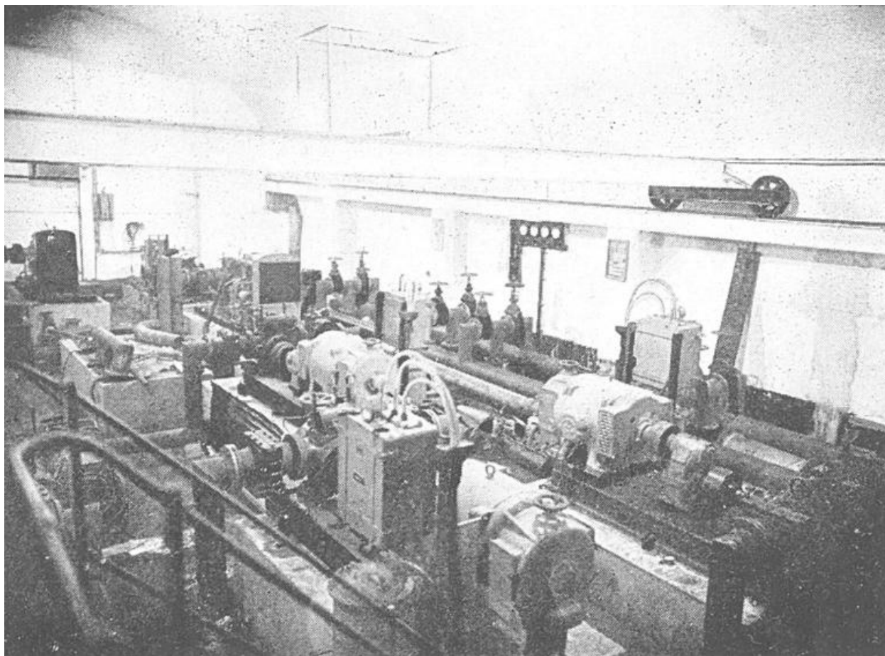
Vue de la salle des pompes dans l'alvéole secondaire, décembre 1953. On voit le chemin de roulement du pont roulant de 10 t
