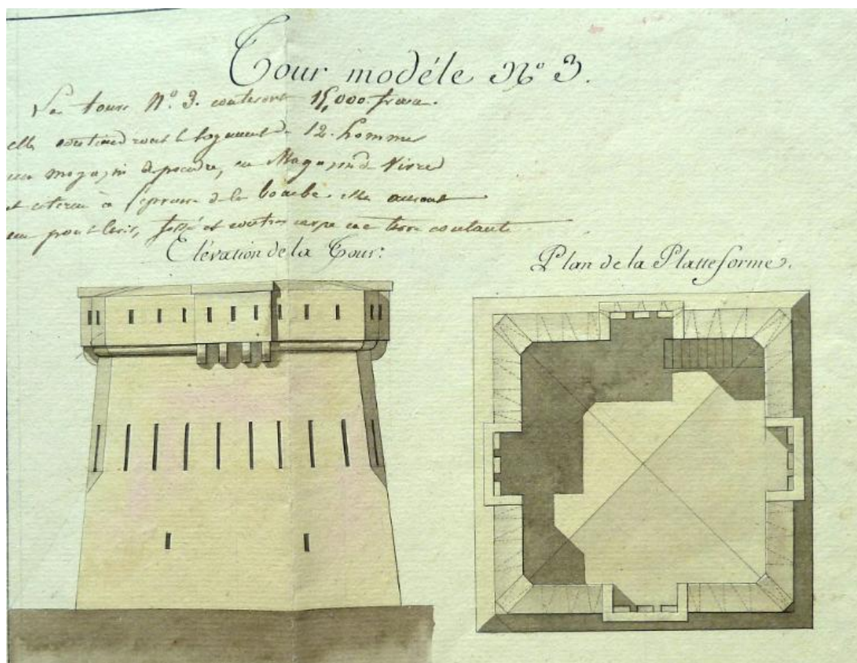
Plans, coupes et élévations des tours-modèles adoptées par sa majesté, 1811 : tour modèle n° 3 (pour 12 hommes)
