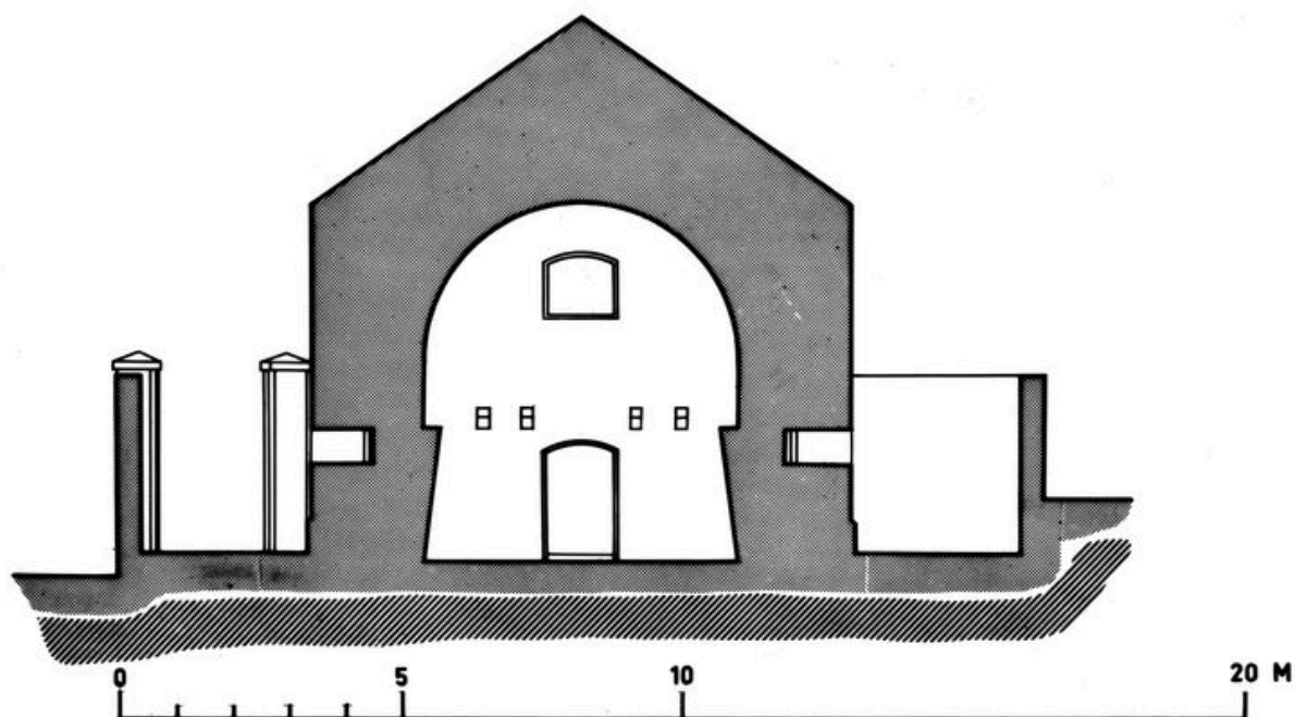
COUPE V.V
