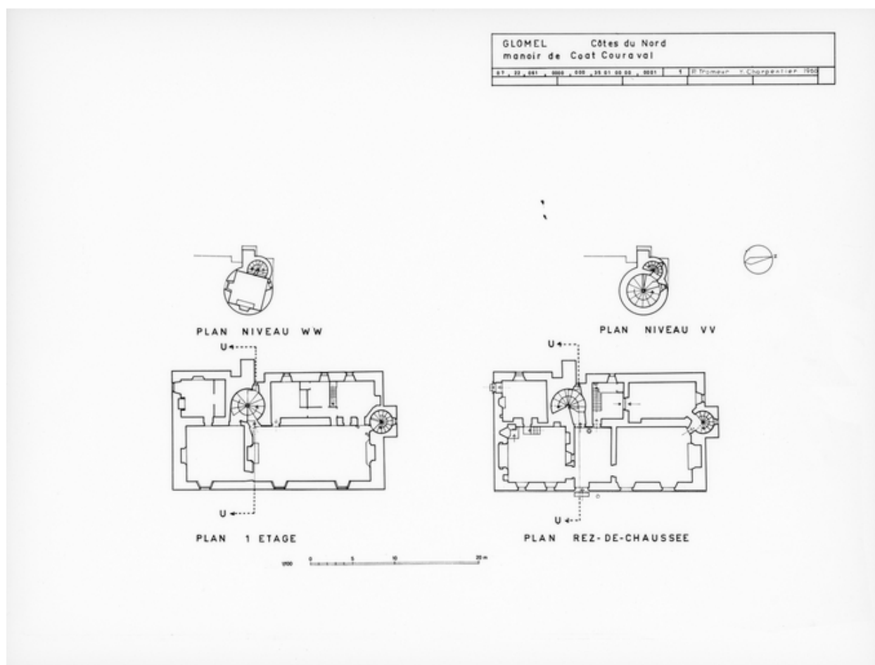
Plans du rez-de-chaussée et du 1er étage
