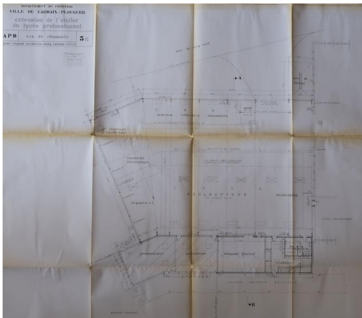
Extension des ateliers du lycée professionnel, plan du rez-de-chaussée (Jean Coignat, architecte, 1989).
