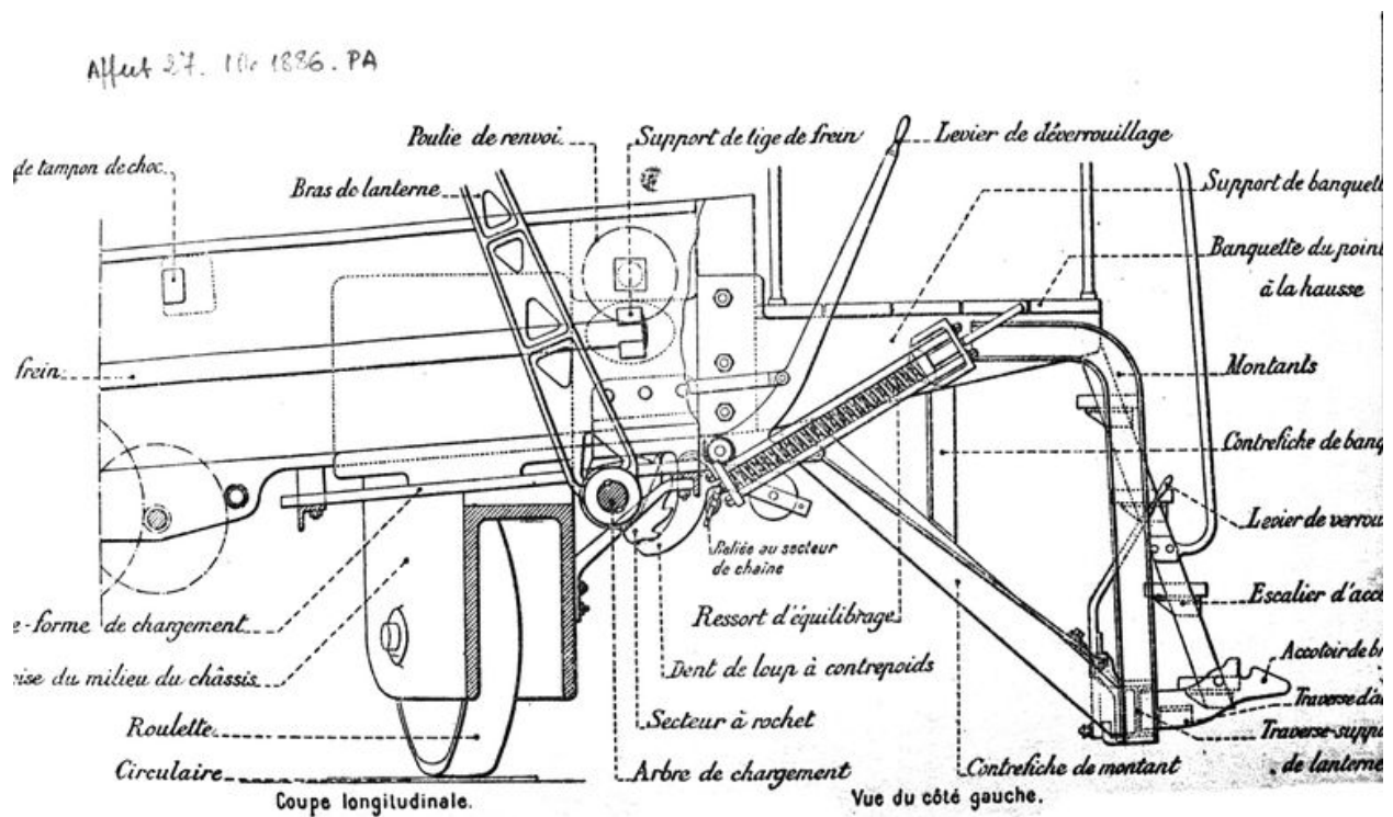
Plan détaillé d'un affût modèle 1886 PA pour canon de 27 cm
