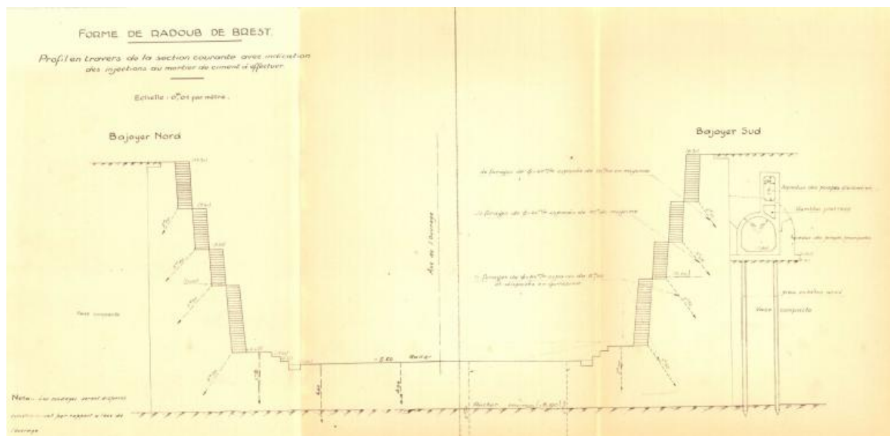
Forme de radoub de Brest : profil en travers de la section courante avec indications des injections au mortier de ciment à effectuer (1948)
