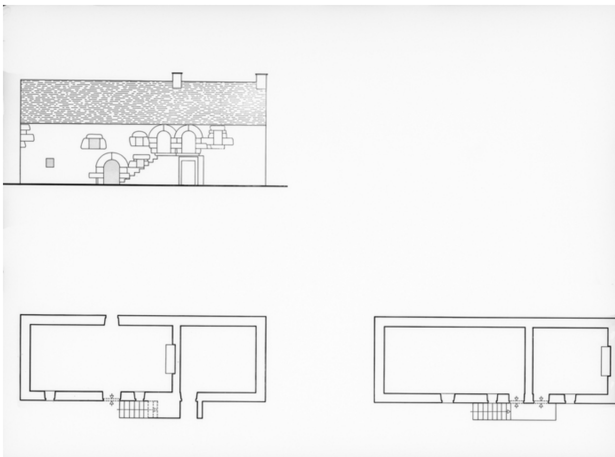
Elévation, plan au sol, plan à l'étage
