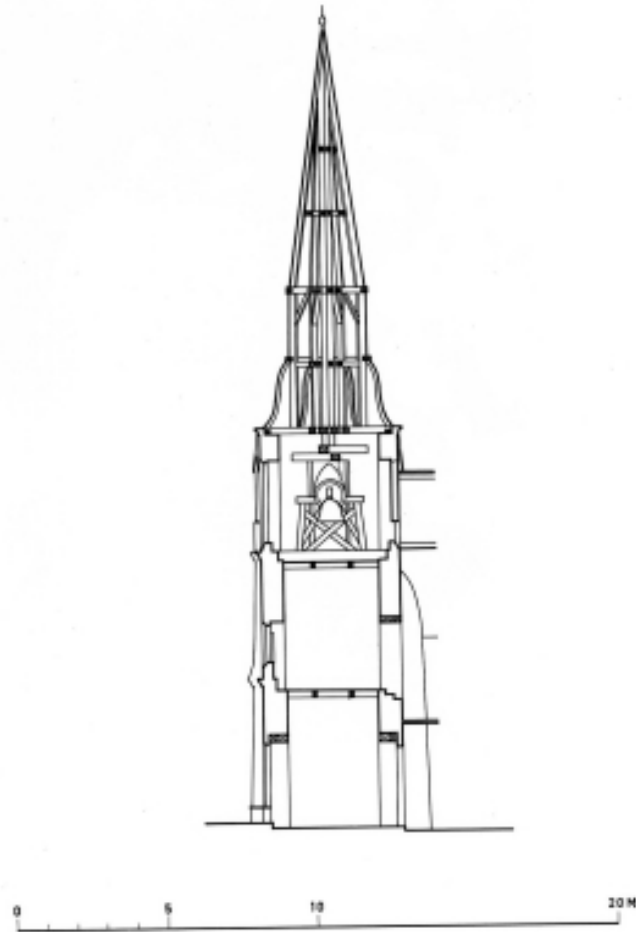
COUPE V V
