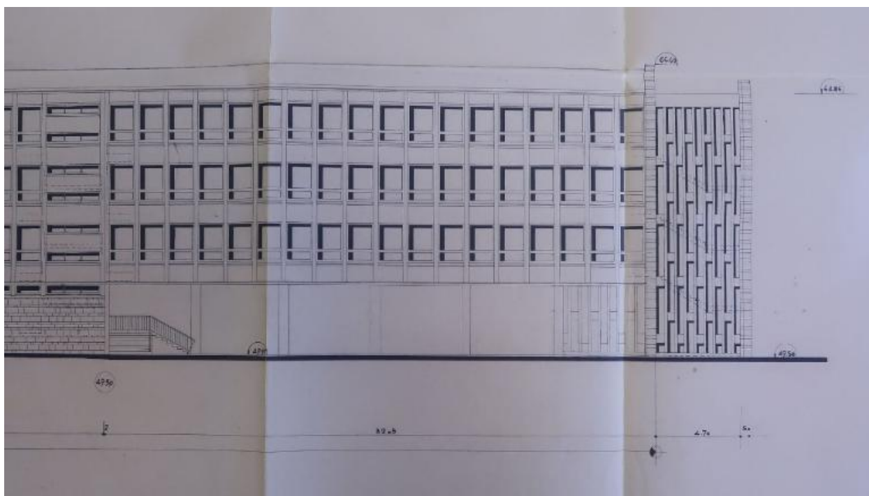
Elévation de la façade ouest. Georges Tourry et Hervé Péron, architectes, 1960.
