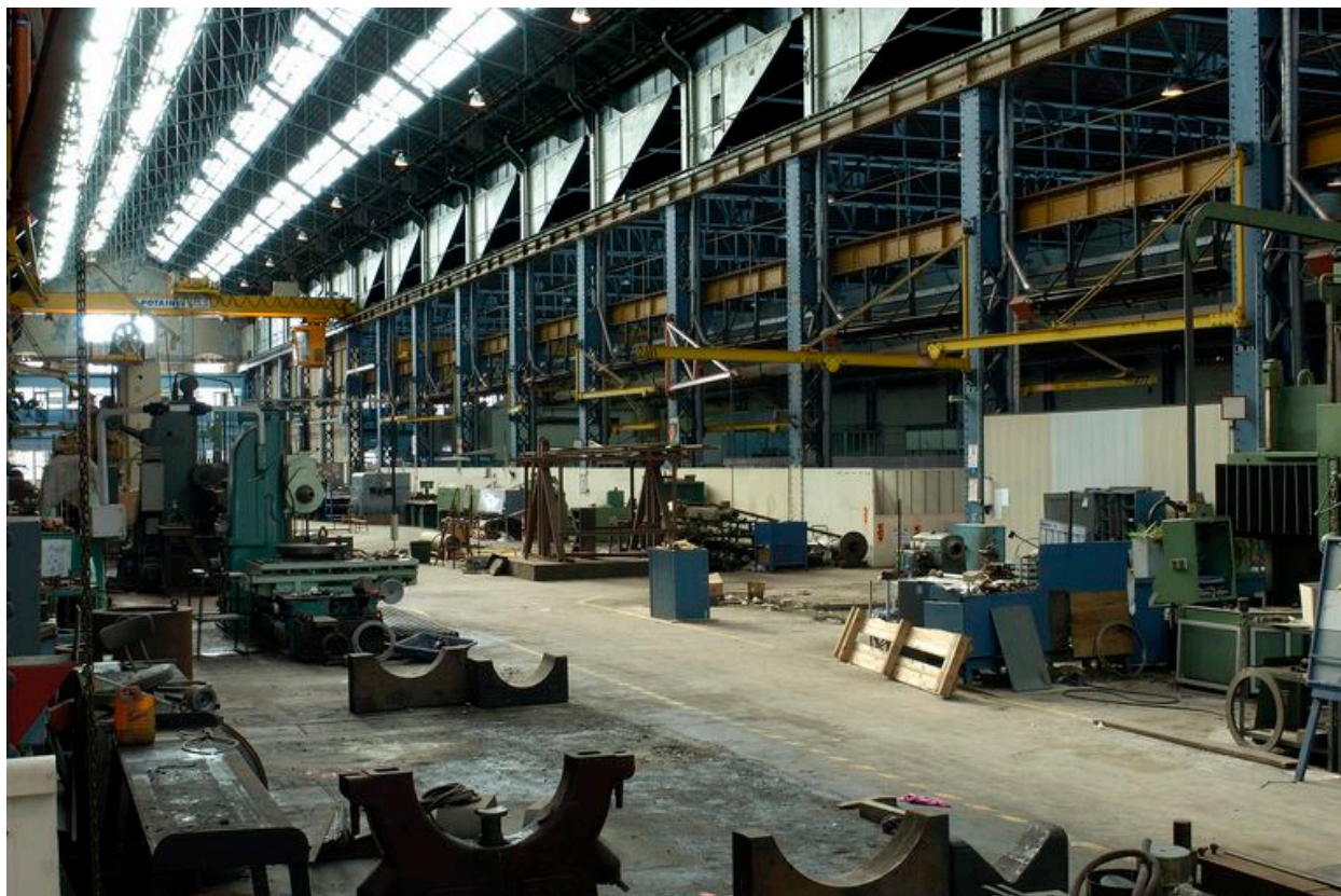
Vue intérieure de la halle d'usinage : un des ateliers annexes couvert de sheds
