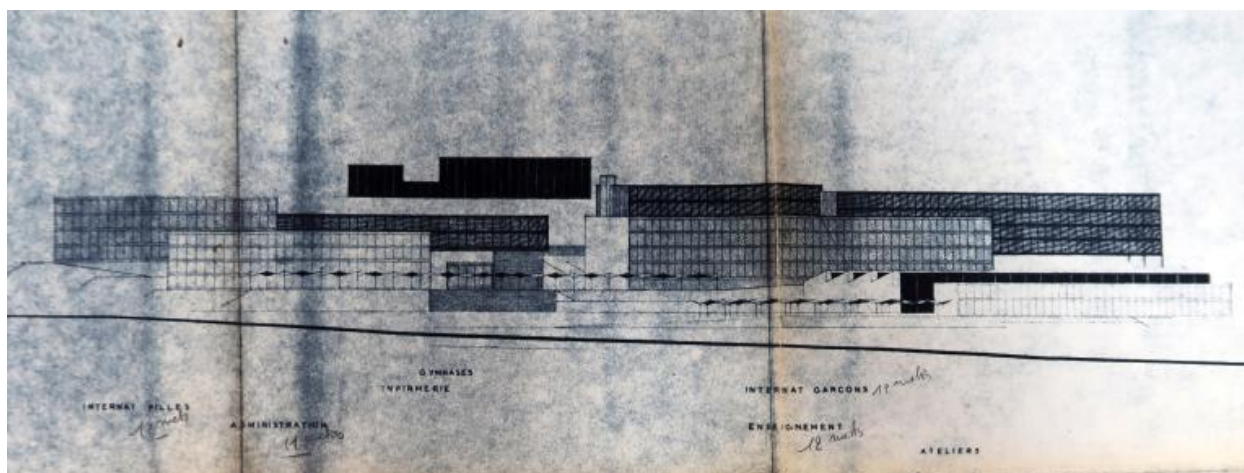
Elévation - Coupes, détail (vue depuis le nord). G. Massé, P. Bigot, F. Roy, J. Monge, M. Doignon-Tournier, architectes, 17 février 1964.
