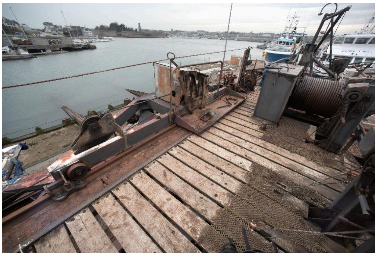
Passerelle : système mécanique
