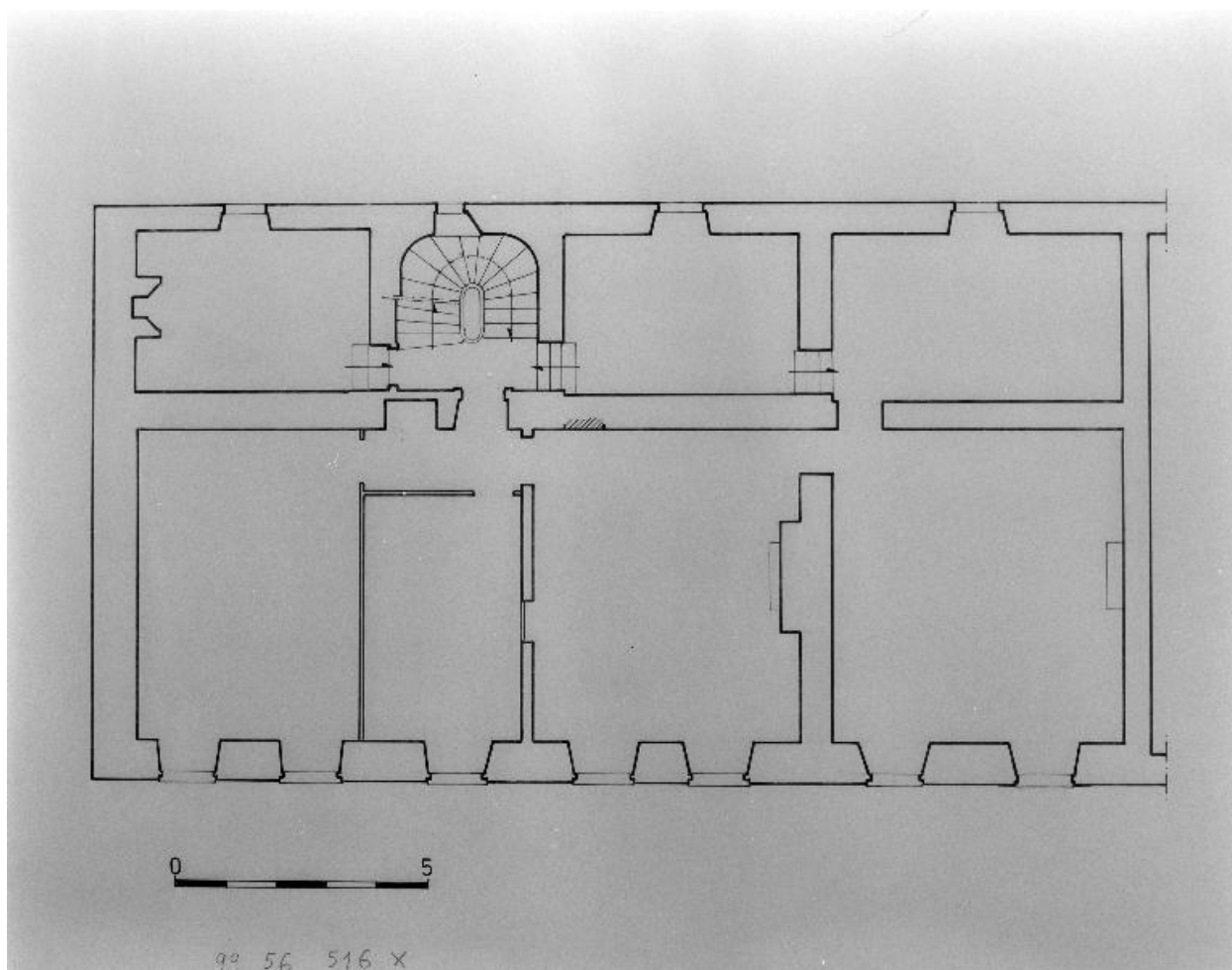
Plan au sol de l'étage.
