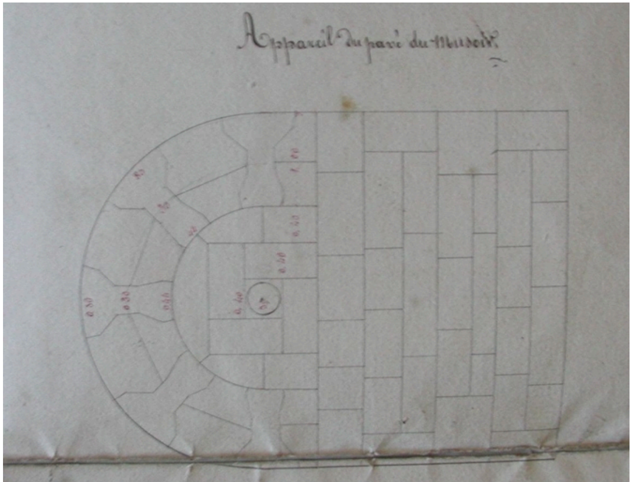
Plan détail : appareil du pavé du musoir, 1852 (AD 22)
