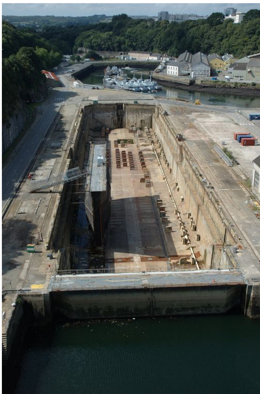
Vue d'ensemble des formes de construction, bassins de radoub actuellement bassins n° 4, 6 et 7 depuis le pont de l'Harteloire : bassin n° 4
