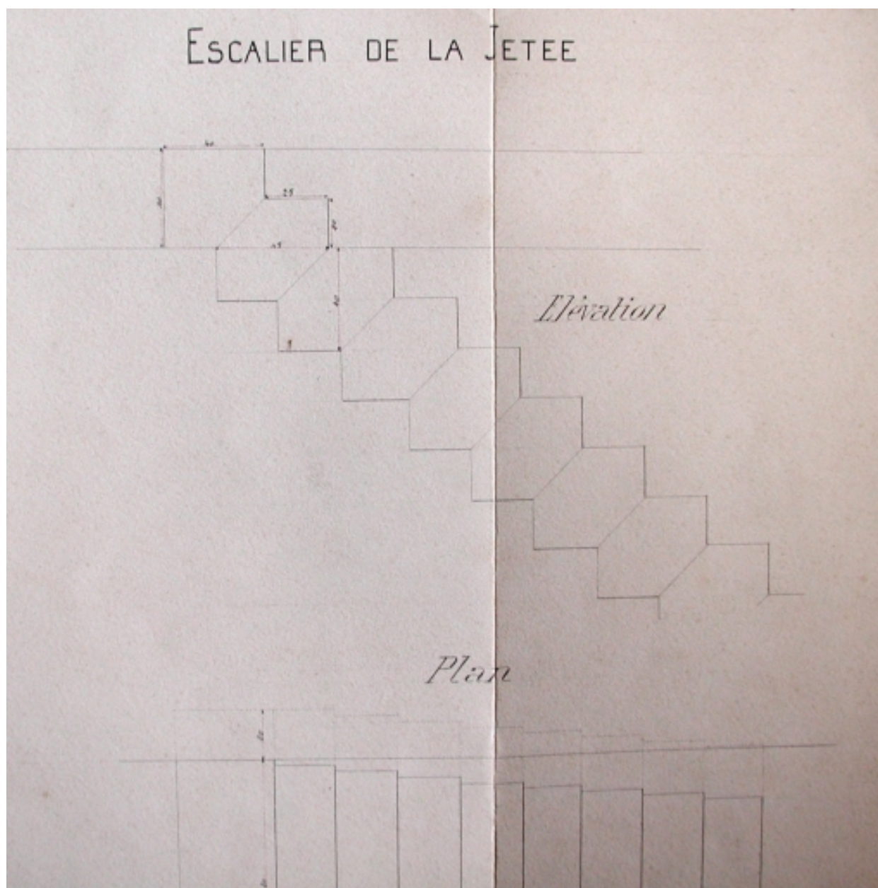
Plan : escalier de la grande jetée de Portrieux, 1860 (AD 22)
