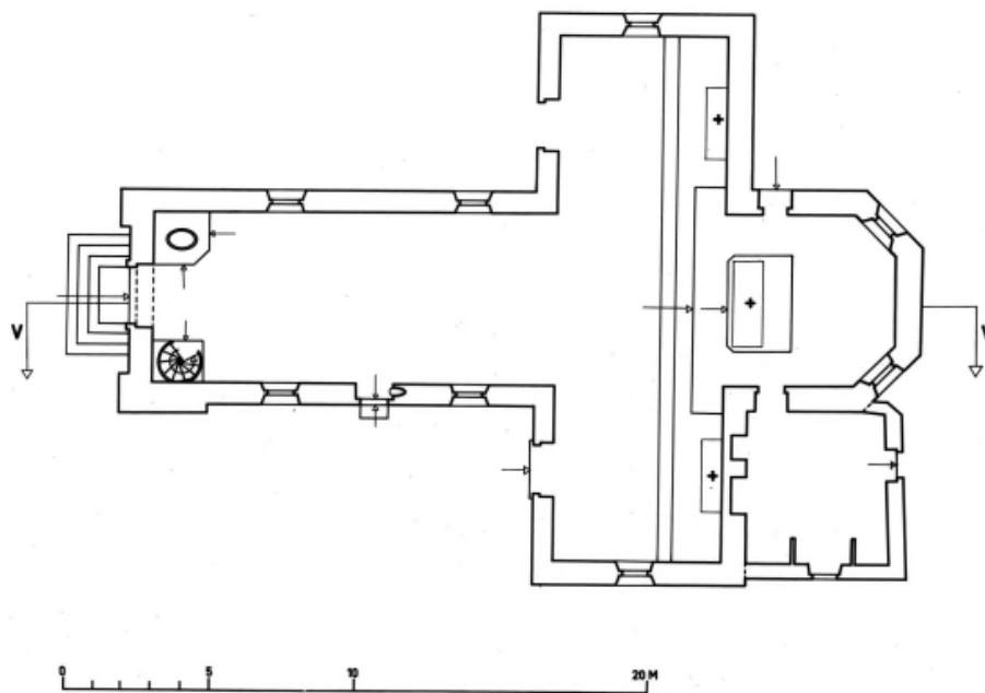
Plan au sol.
