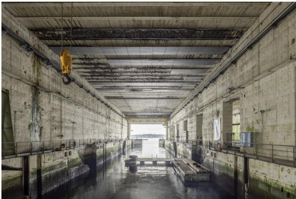
Vue générale de l'alvéole G (n° 13 et 14) en eau
