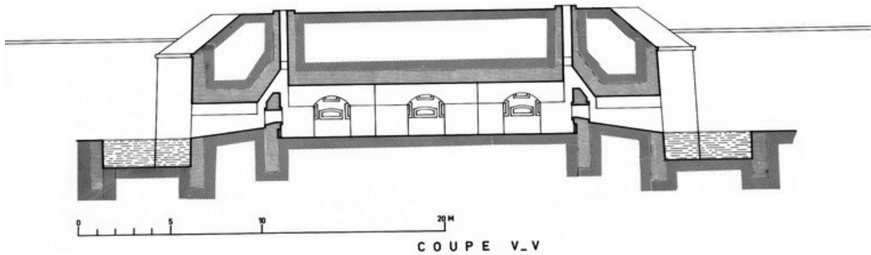
Coupe V-V de la caponnière Ouest (D) (Lecoq)
