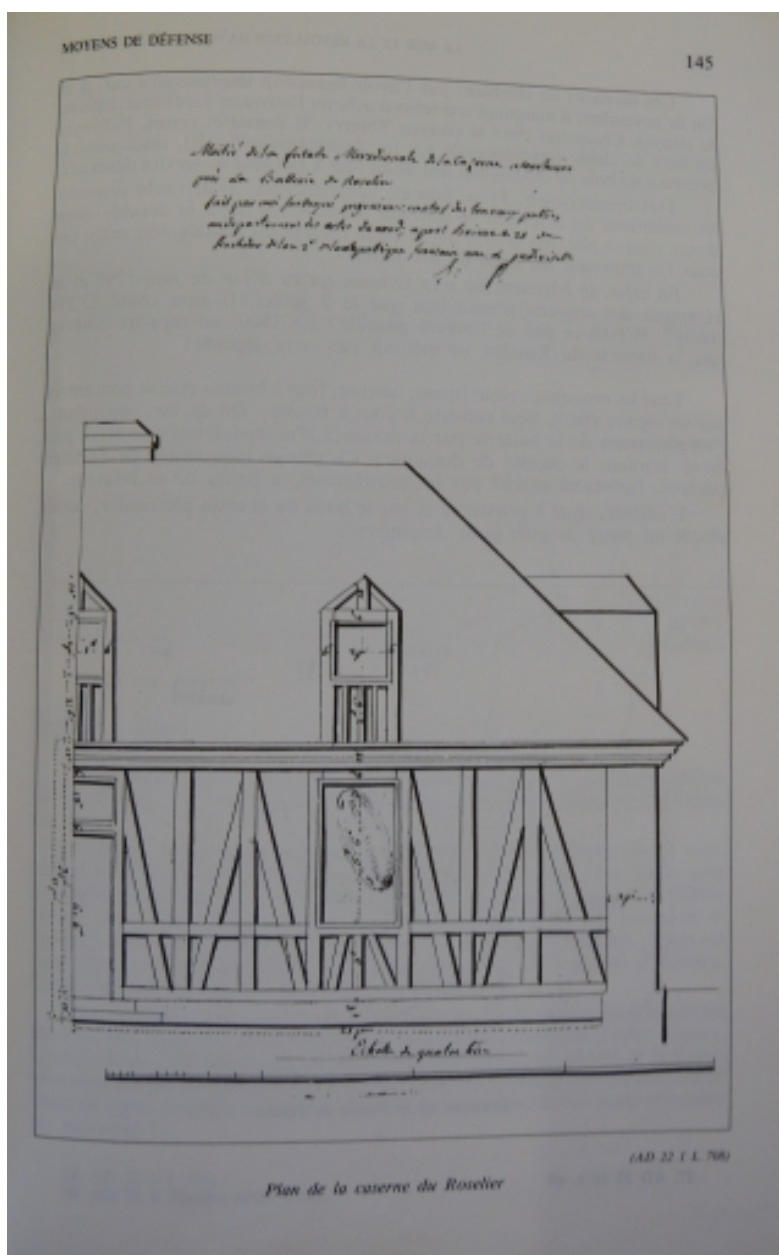
Plan de la caserne du Roselier (Sallier Dupin, Guy, AD 22, 1 L 708)
