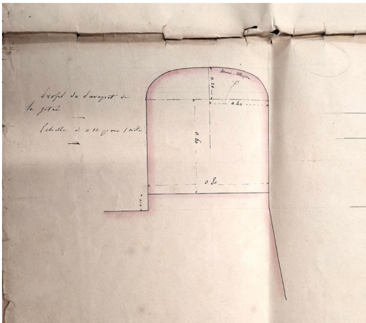
Profil du parapet de la jetée du phare de la pointe de l'Aigle (7 novembre 1855)
