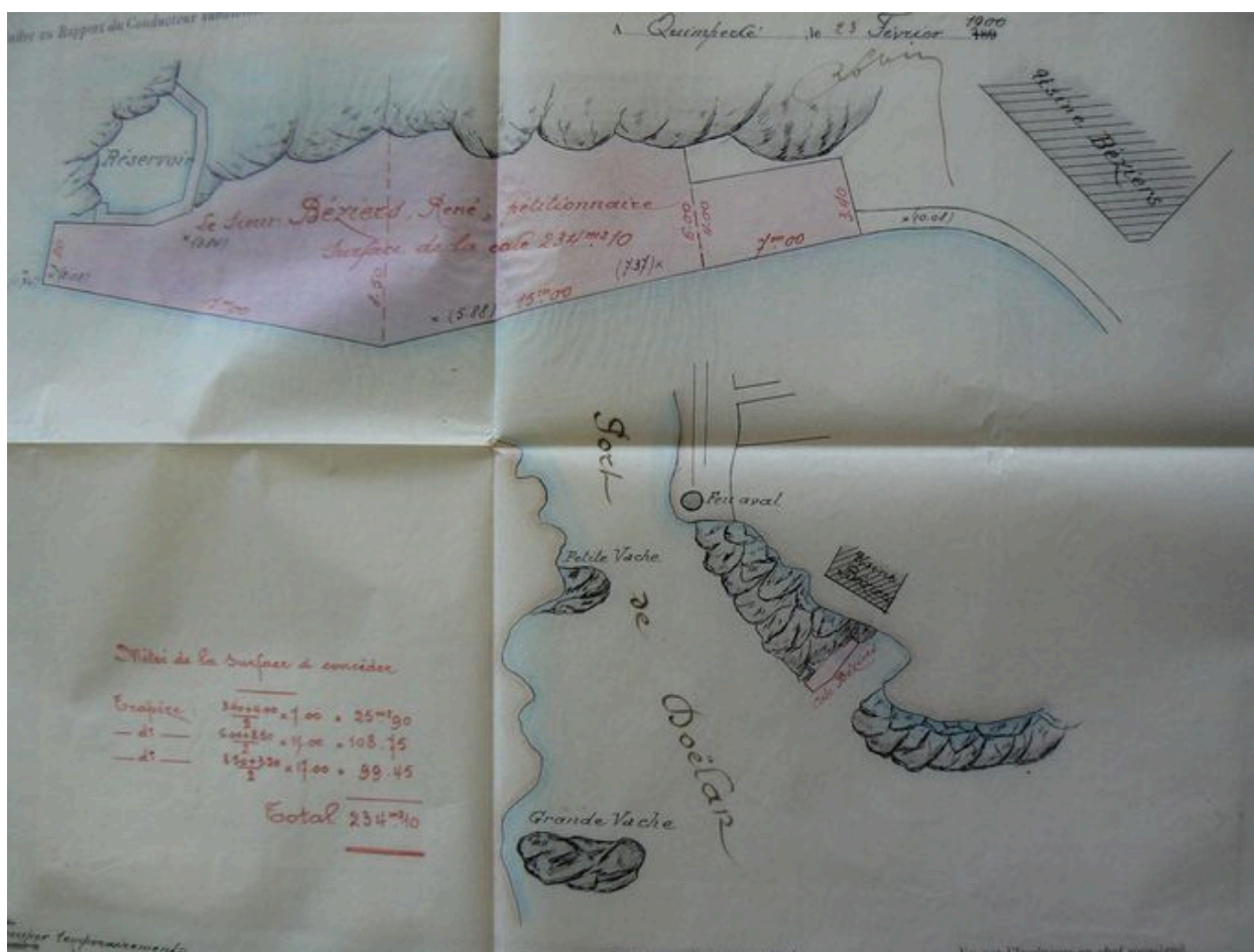
Plan de la cale Cayenne, réalisé par les Ponts-et-Chaussées
