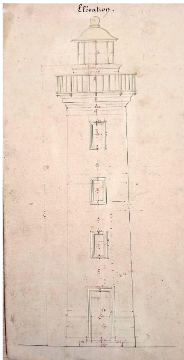
Elévation du phare de la pointe de l'Aigle (29 novembre 1851)
